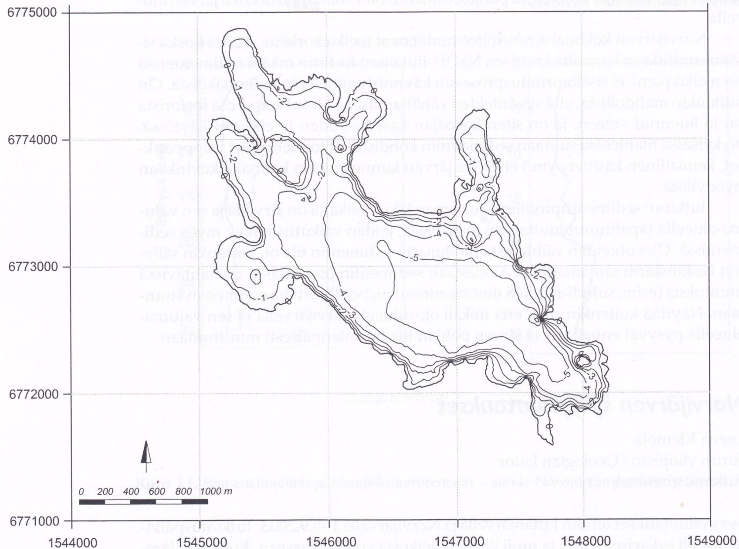
Kuva 22. Narvijärven syvyyskartta.
